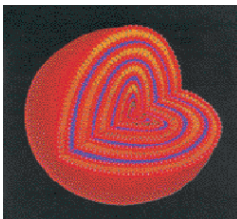
Sphérulite
